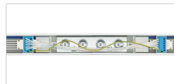
Sehr stabile Kupplung zwischen den Tragschienen für lange Abhängeabstände von bis zu 4,6 m
