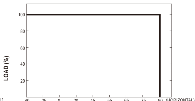
Tcase (°C)
