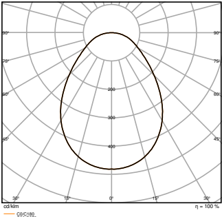
DL SLIM ALU DA D280 V 25W MS 840 WT
