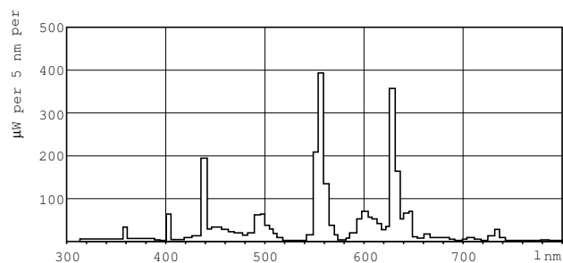
Lichtfarbe /840
